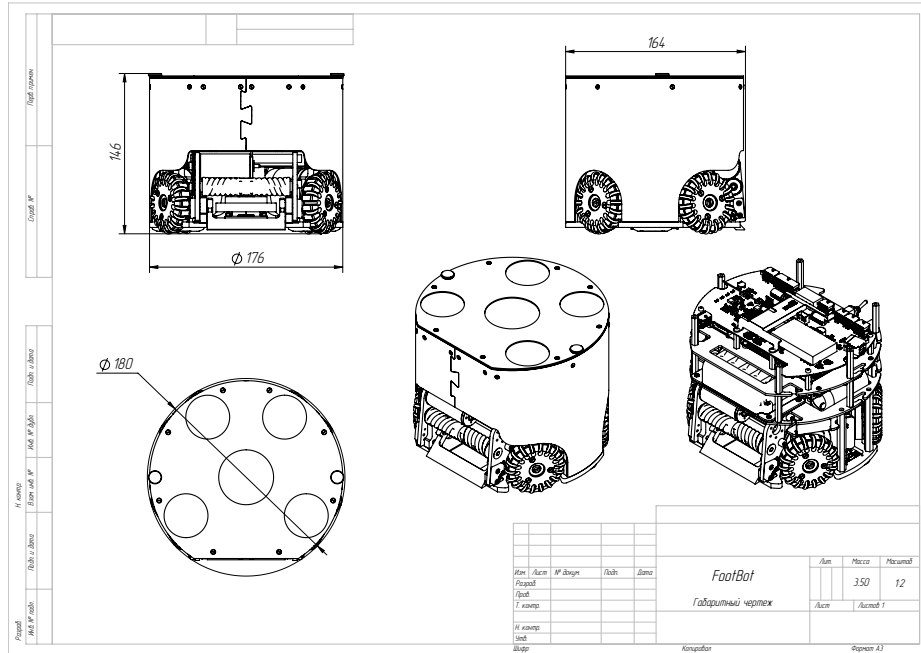
Рис. 1: Чертеж робот
