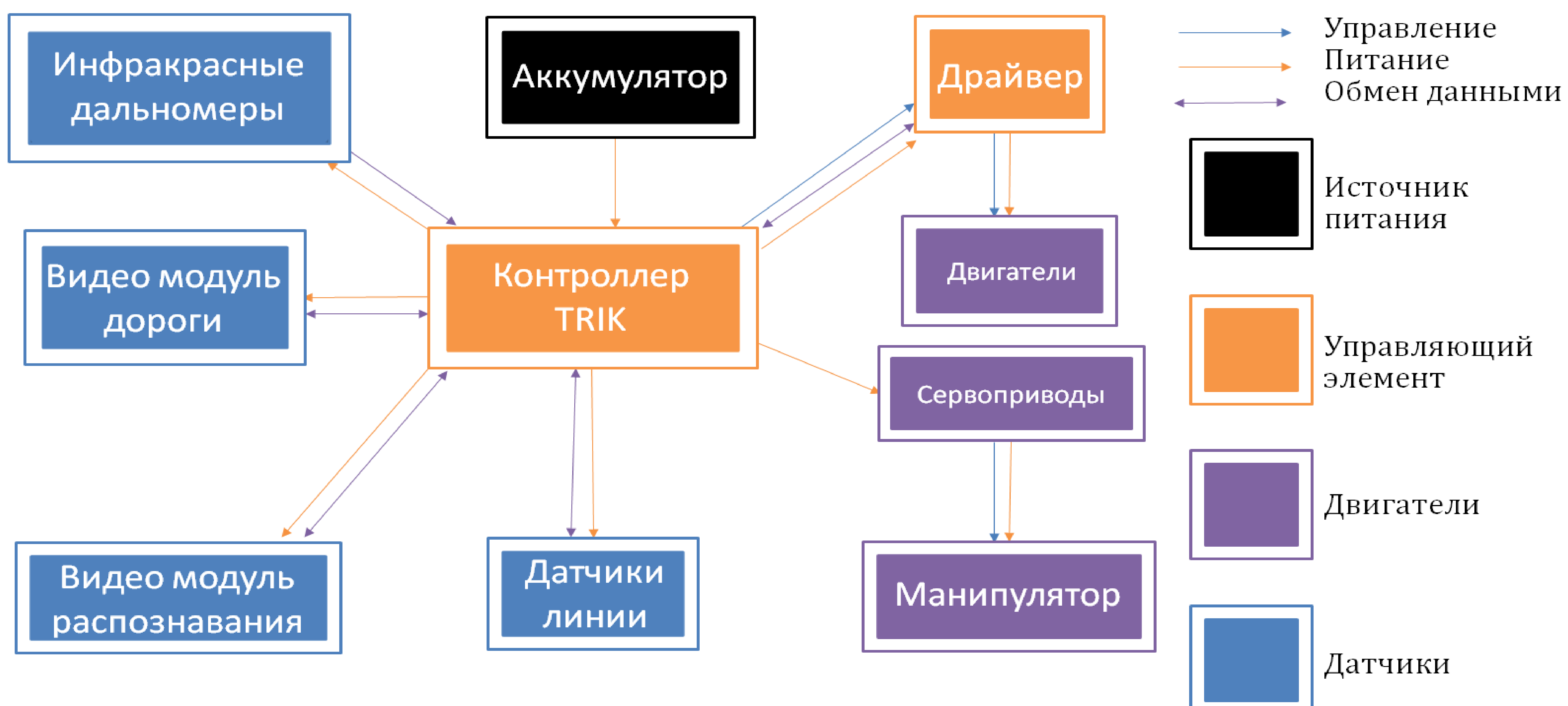
Функциональная схема
