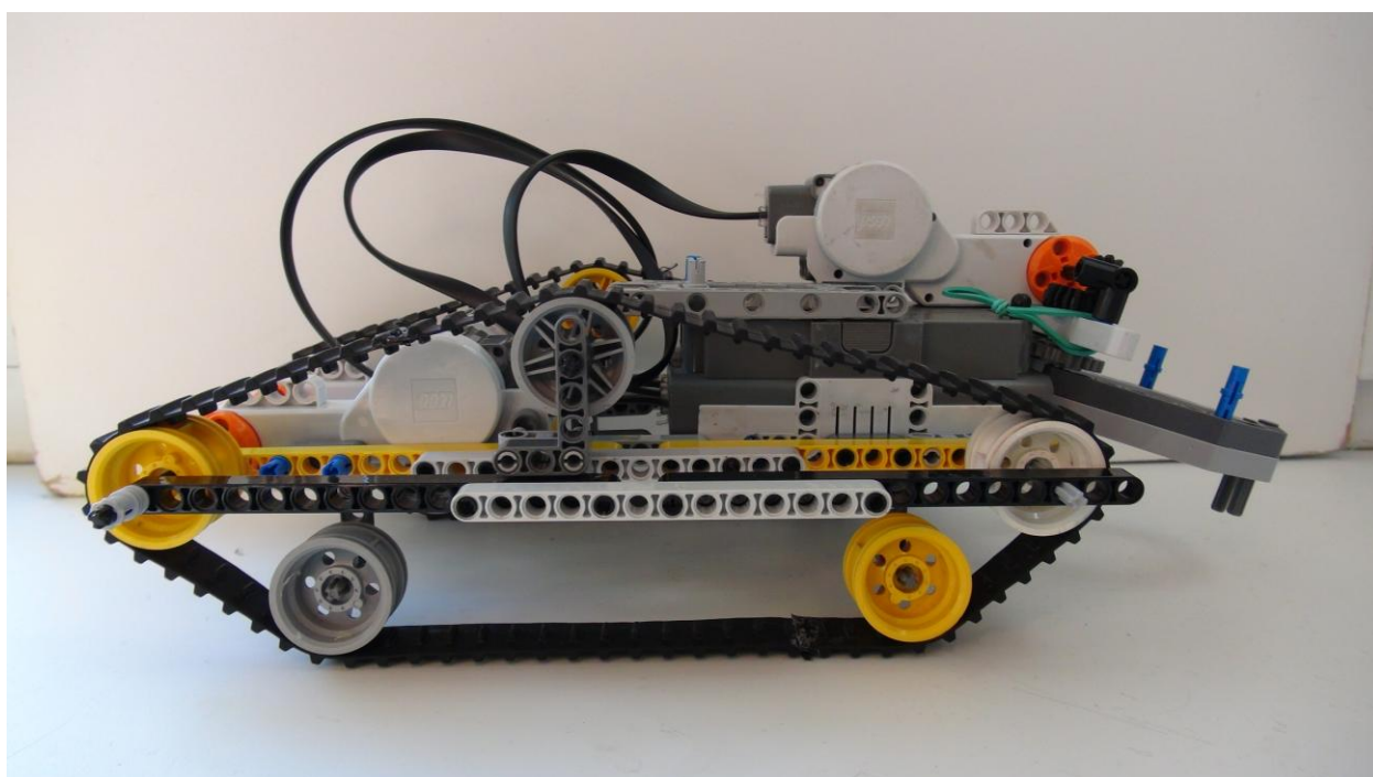
Вид сбоку
