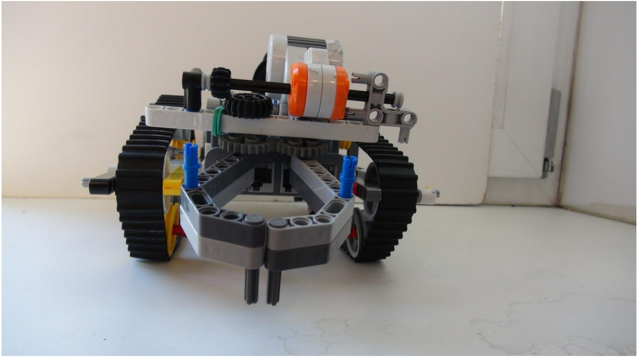
Вид спереди
