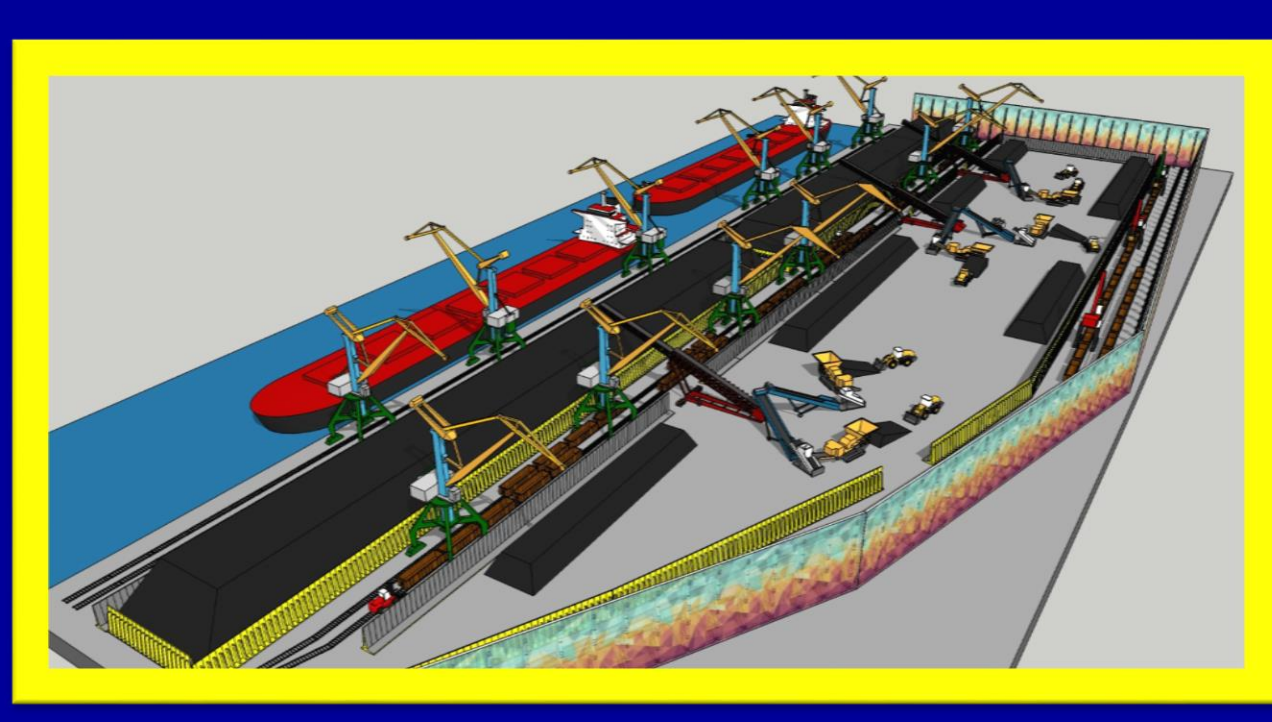
Схема погрузки навалочных грузов до реализации проекта
